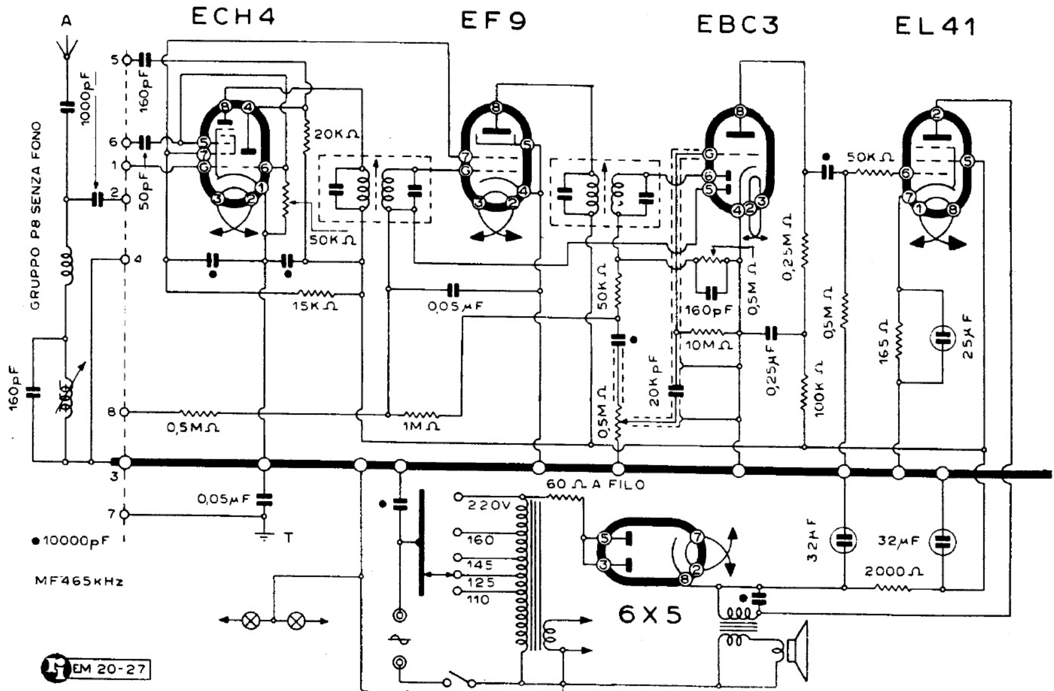
NOVA RADIO - Mod. A2
